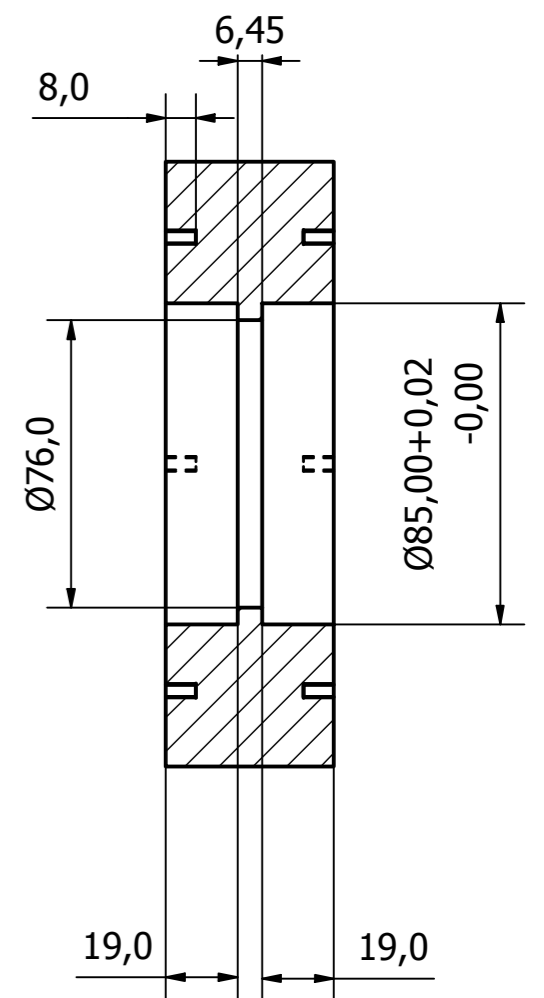
A-A (1 : 2)
